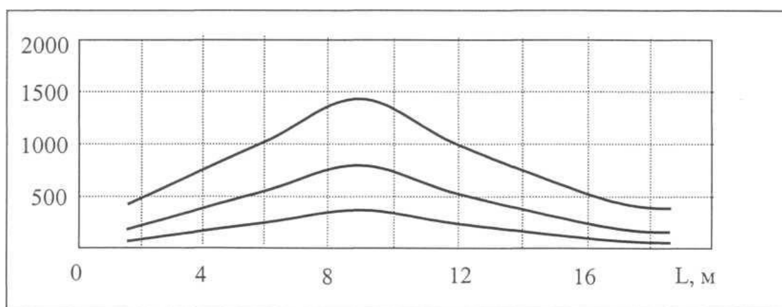
Рис. Зависимость плотности теплового потока Q при горении зданий и сооружений
