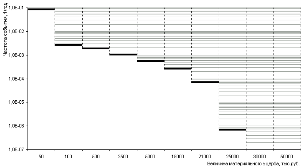
Рис. Диаграмма риска материальных потерь (F/G) при авариях на взрыво- и пожароопасных опасных объектах
